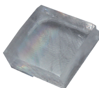
方解石
