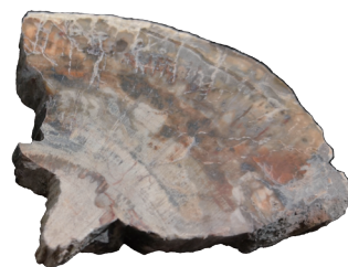
珪化木
