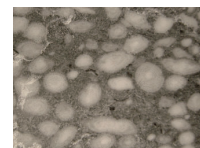
フズリナ石灰岩
